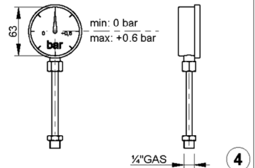
MANOMETRO PRESSURE GAUGE
