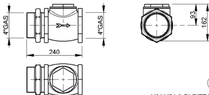
VALVOLA DI RITEGNO NON RETURN VALVE tipo-type: VR15
